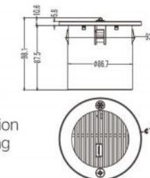
L-7023 Vent Grille
