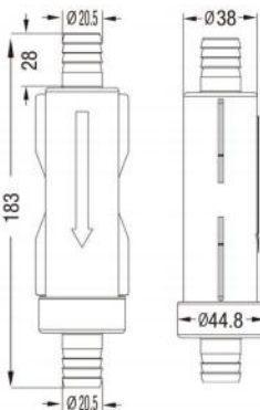
L-2220 Ozone Mixer
