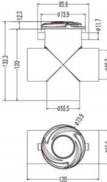
L-2047 1.5" Xiongfeng Diverter Values Black
